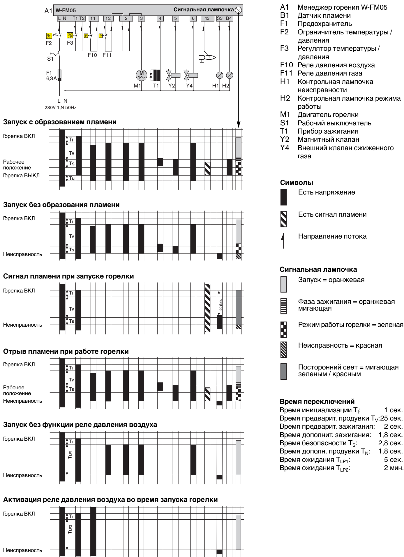
Диаграмма последовательности выполнения функций
