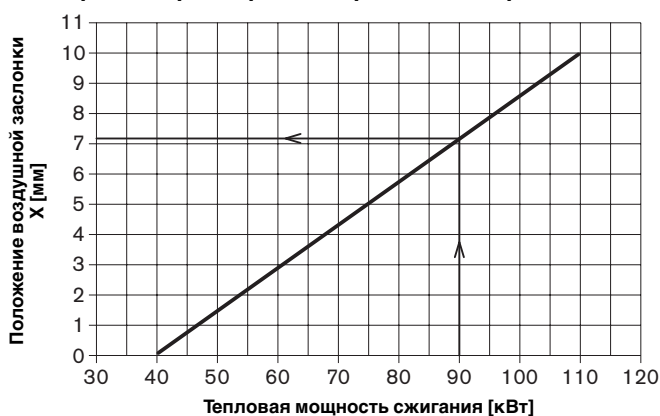
Диаграмма предварит. настройки подпорной шайбы
