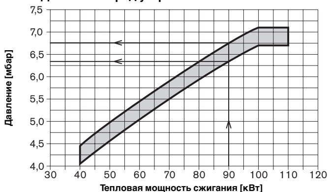
Давление перед устройством смешивания
