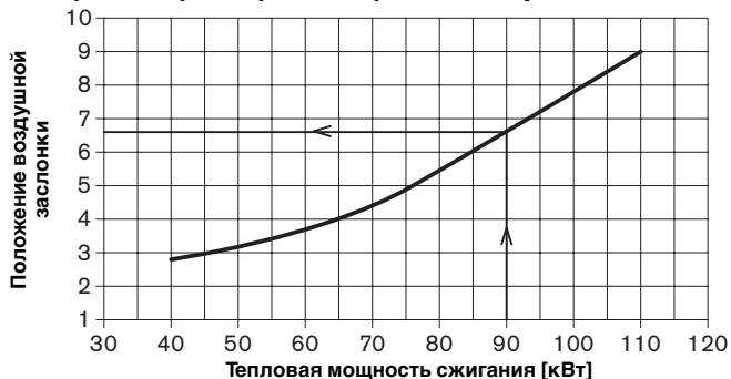
Диаграмма предварит. настройки воздушной заслонки
